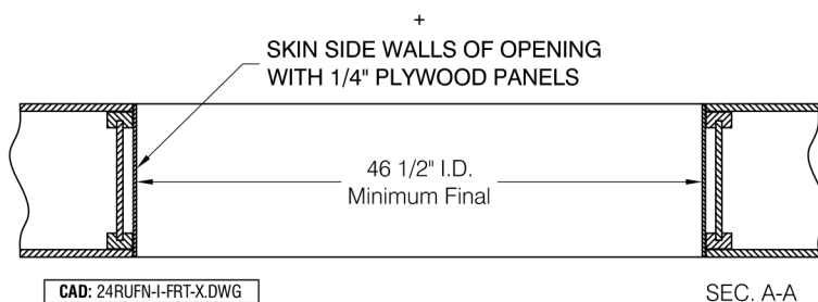
SEC. A-A
